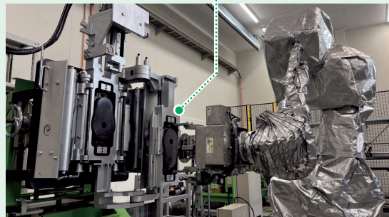
REX-ROBO®による交換作業
